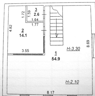
Литер Б мансарда
