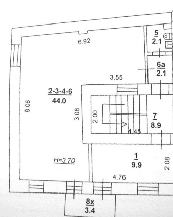
Литер Б 2 этаж
