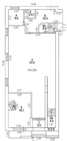
1 этаж
