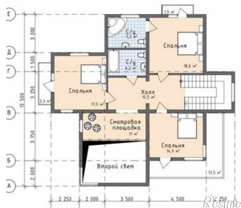
План с расстановкой мебели и оборудования на отм. +3,200
