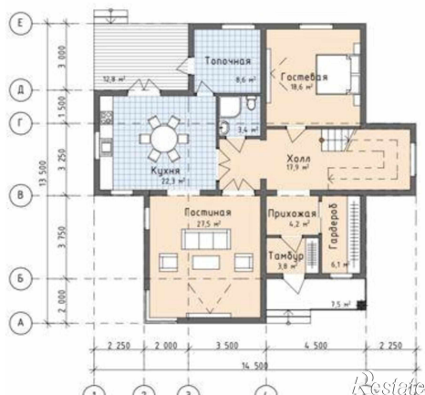
План с расстановкой мебели и оборудования на отм. 0,000
