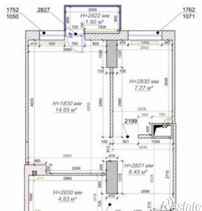
Обмерный план
